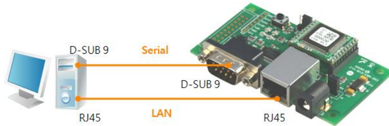
图 2-1 为了试动作与PC连接
