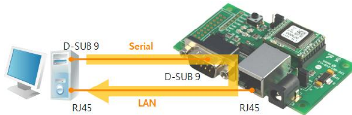
图 2-9 RS232 → LAN
