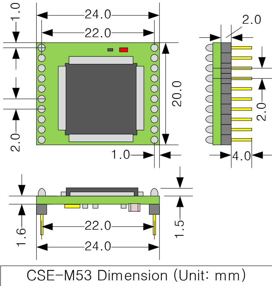
图 1-5 CSE-M53 规格
