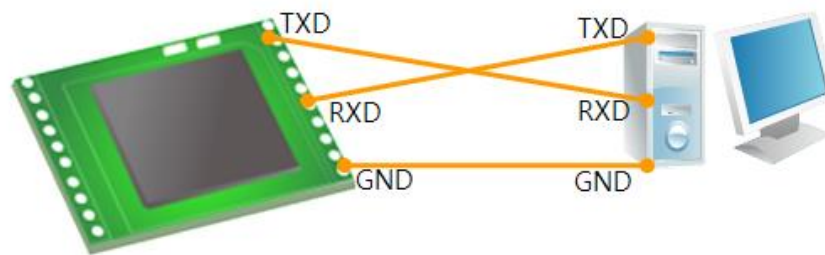
图 8-1 正确的RS232连接
