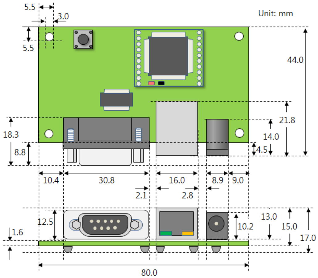
图 1-10 CSE-M53 开发用板规格
