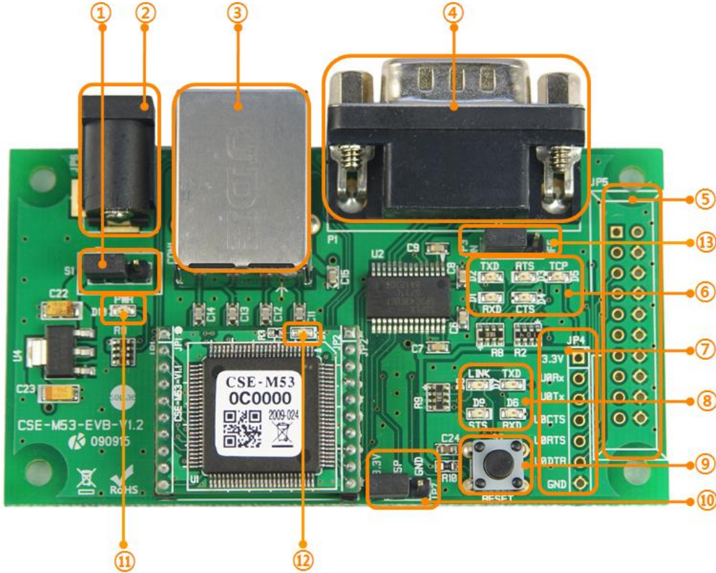
图 1-7 CSE-M53 开发板
