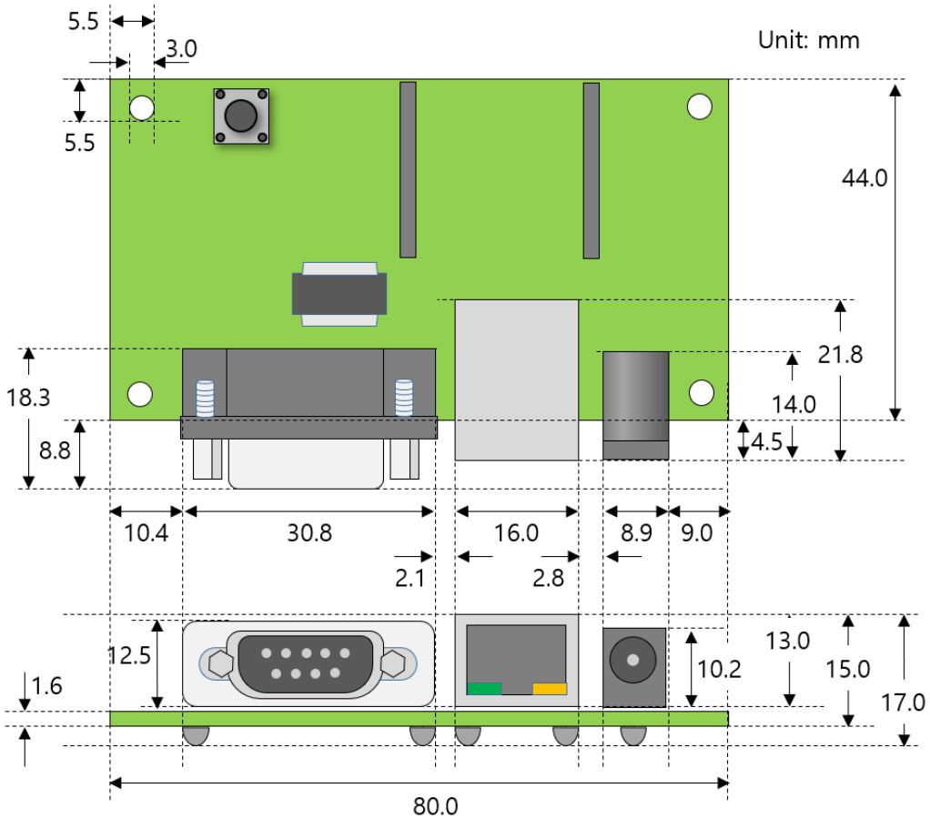
그림 1-5 CSE-M53/M53N-EVB2 치수
