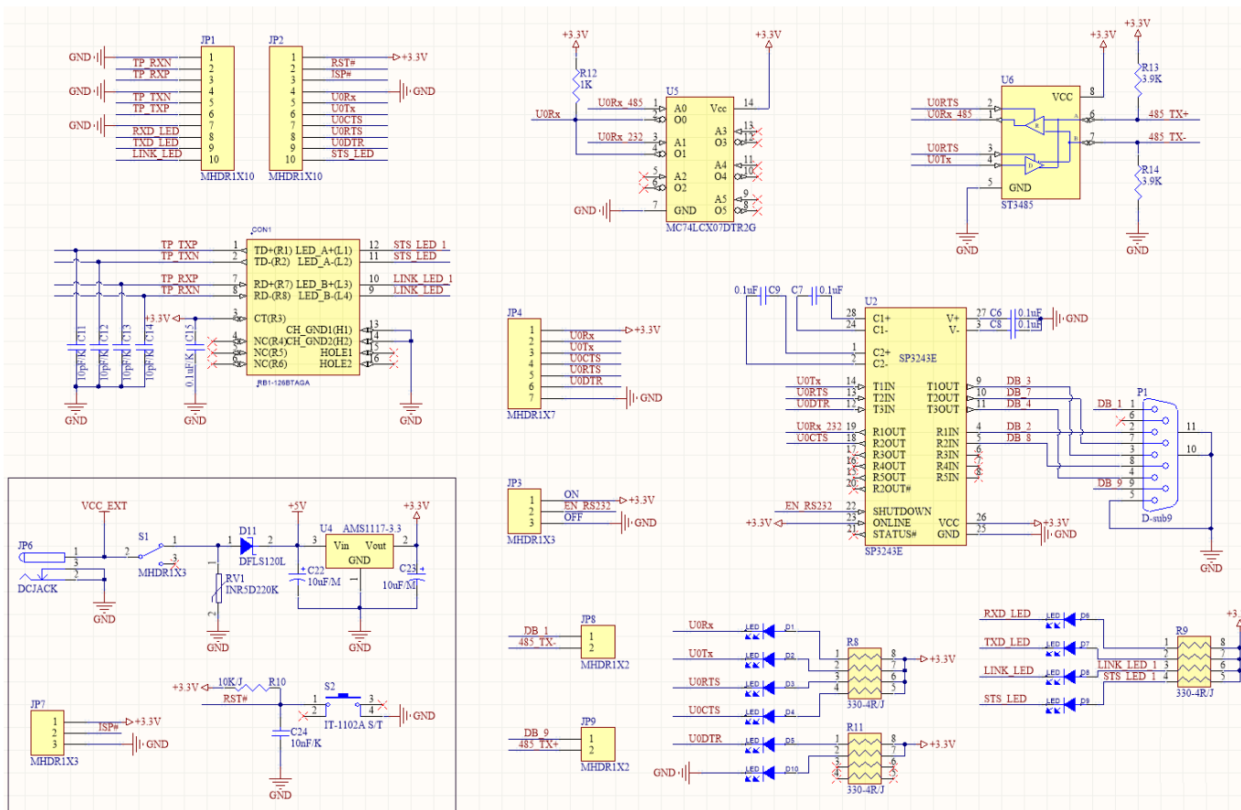
그림 1-1 CSE-M53/M53N-EVB2 회로도
