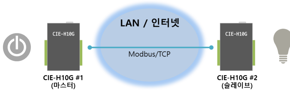
그림 1-3 1:1 인터넷 스위치 구성
