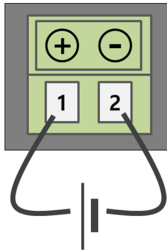
그림 1-8 전원입력 방식
