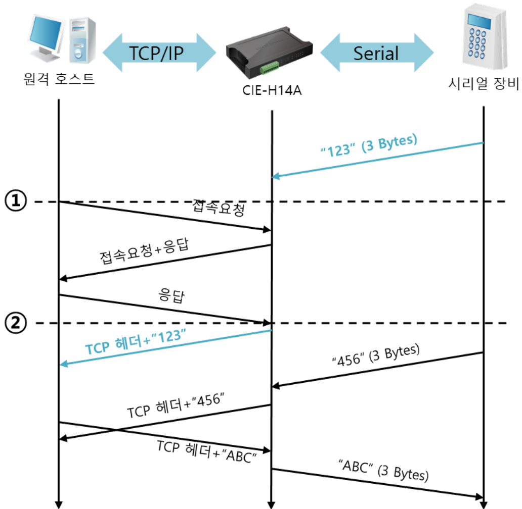
그림 6-2 접속 전 데이터 크기가 1인 경우
