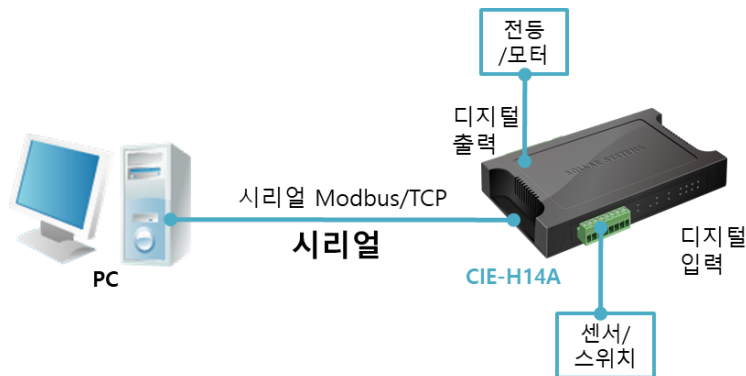
그림 1-2 시리얼 Modbus/TCP 구성 예
