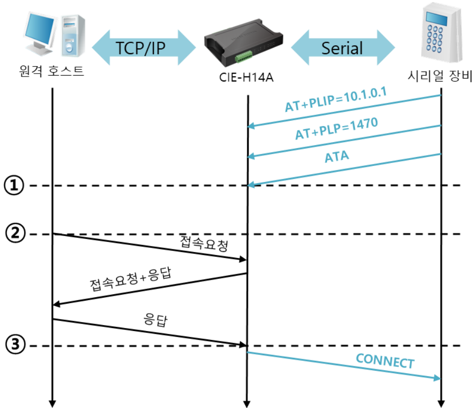
그림 6-7 TCP 수동접속
