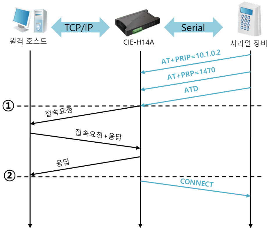
그림 6-8 TCP 능동접속
