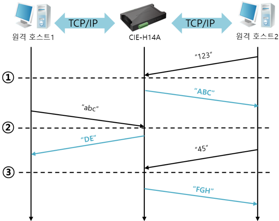
그림 6-11 UDP 동적 호스트 전송
