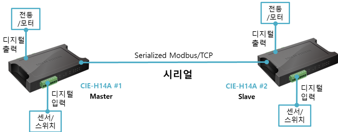
그림 1-4 시리얼 스위치 구성 예
