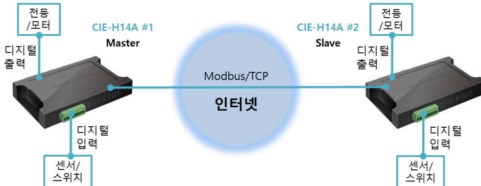
그림 1-3 인터넷 스위치 구성 예
