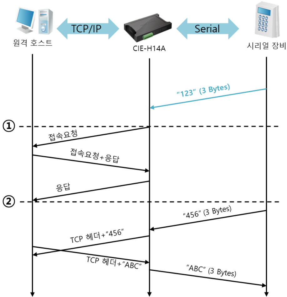
그림 6-4 접속 전 데이터 크기가 0인 경우
