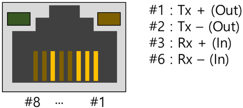
그림 1-13 RJ45 이더넷 커넥터 사양
