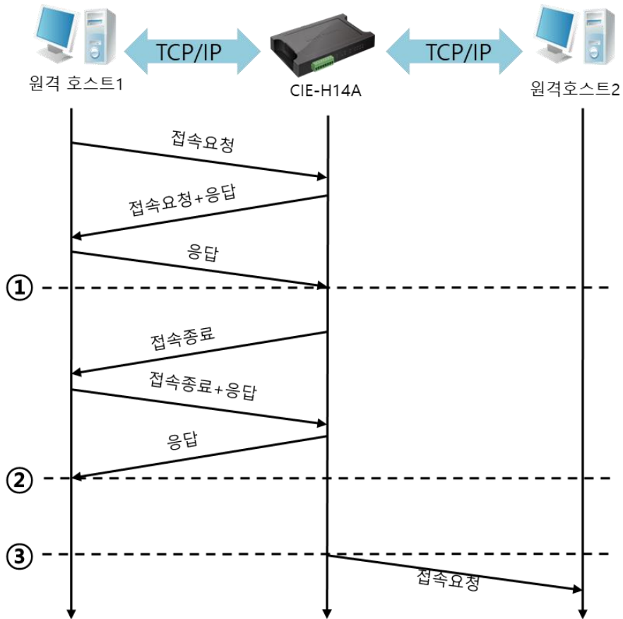
그림 6-6 TCP 서버/클라이언트 모드의 경우
