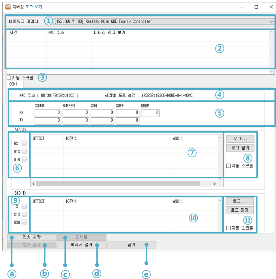
그림 8-4 디버깅 로그 보기 창
