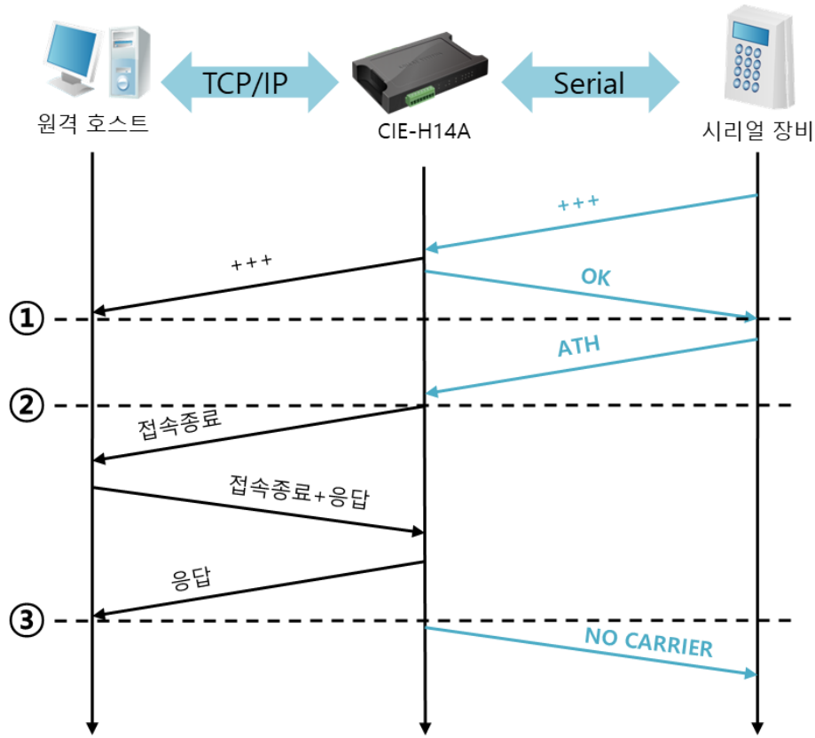
그림 6-9 TCP 접속종료
