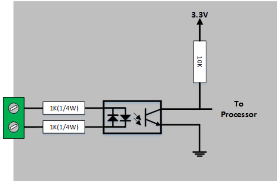
그림 1-9 입력 포트 회로도
