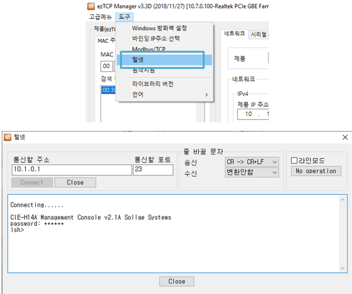
그림 7-5 텔넷 로그인 화면 (ezManager)
