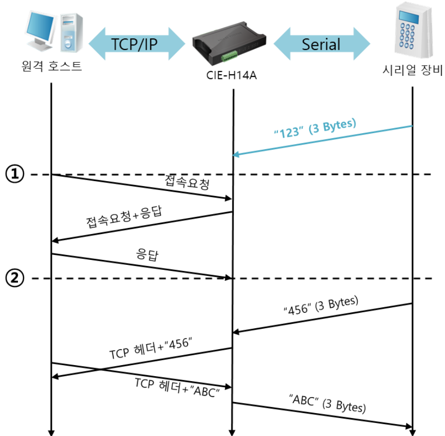
그림 6-1 TCP 접속 전 데이터 크기가 0인 경우
