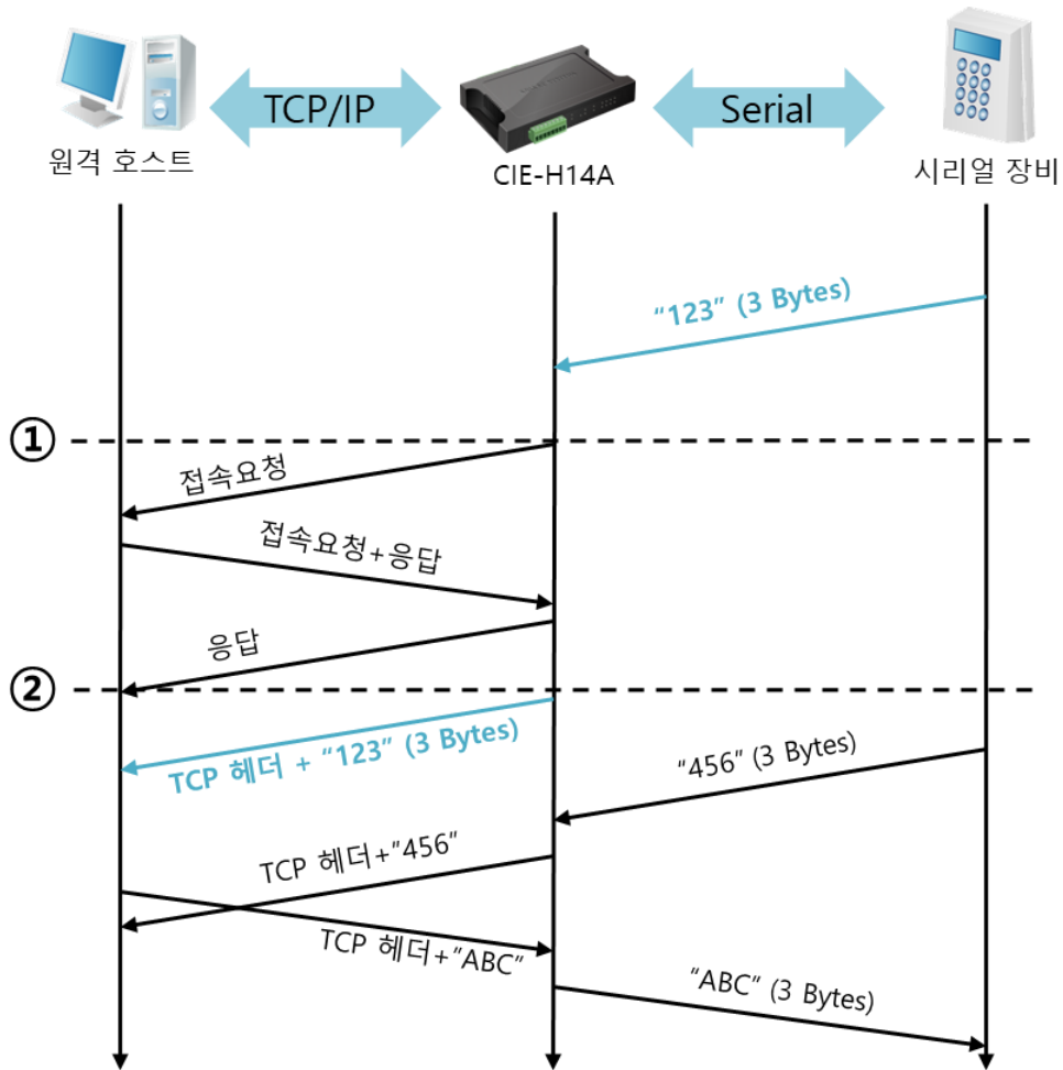
그림 6-5 접속 전 데이터 크기가 1인 경우
