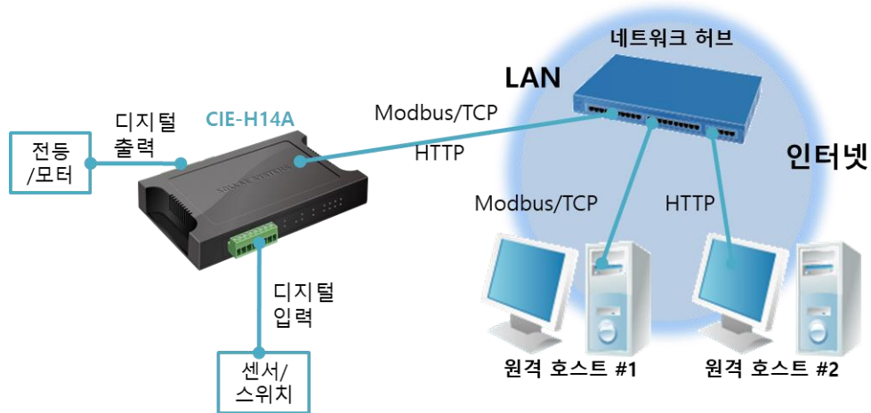
그림 1-1 원격 디지털 입/출력 감시/제어 구성 예
