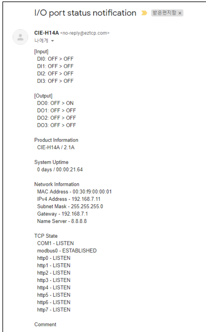
그림 8-7 e-mail 알림
