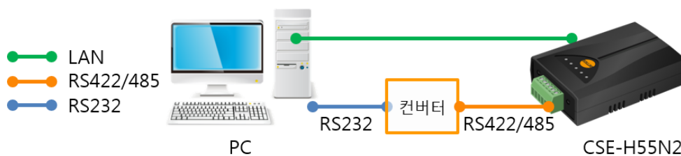
그림 2-1 시험작동을 위한 PC와의 연결
