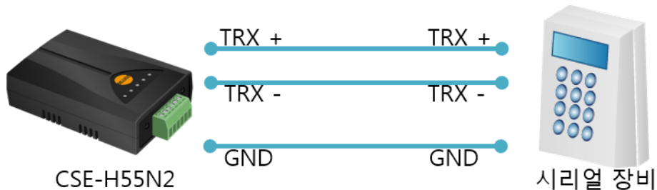
그림 10-1 올바른 RS485 연결
