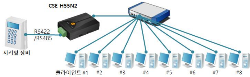
그림 1-7 멀티 모니터링 구성 예
