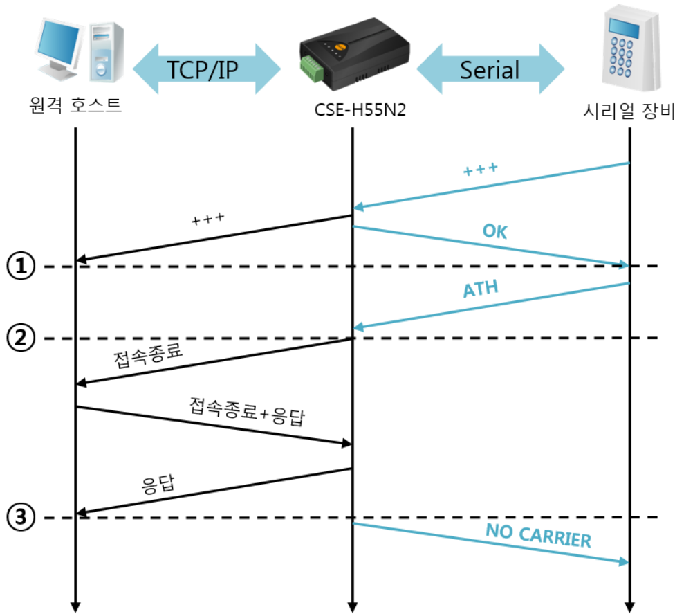
그림 5-9 TCP 접속종료
