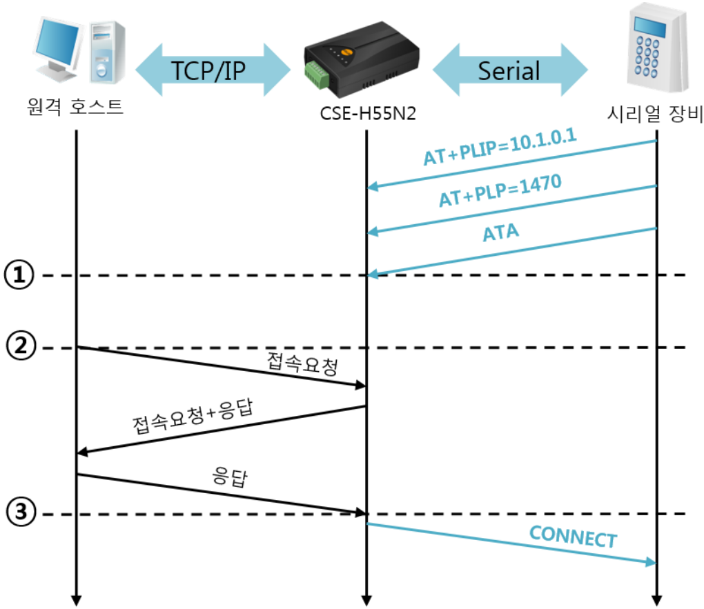
그림 5-7 TCP 수동접속
