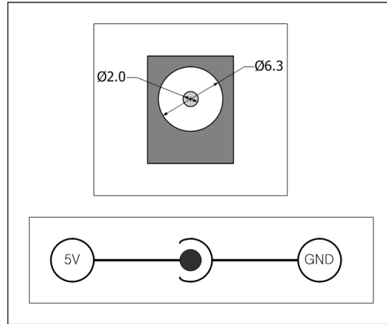
그림 1-9 DC 5V 전원 잭
