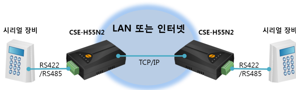
그림 1-5 시리얼 터널링 예
