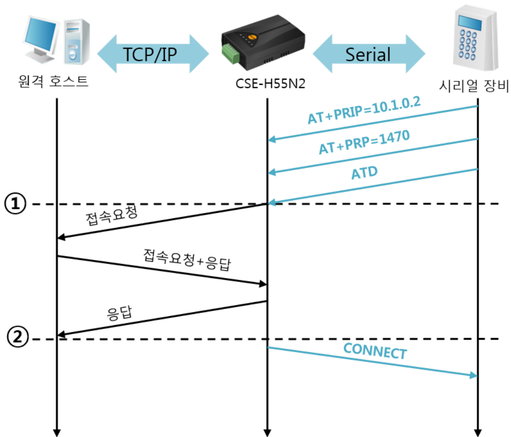
그림 5-8 TCP 능동접속
