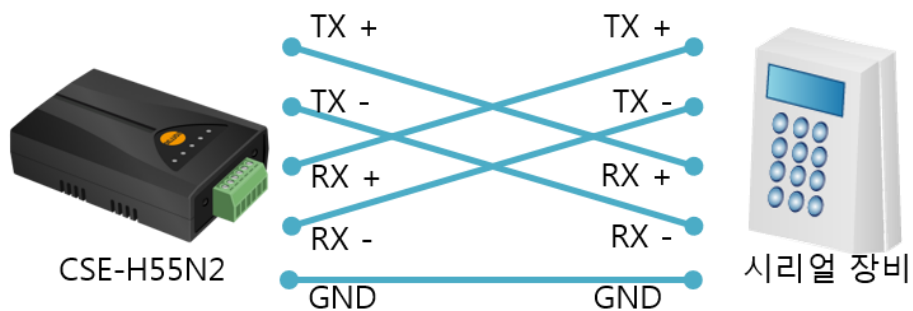
그림 10-2 올바른 RS422 연결
