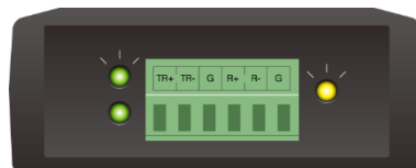
그림 1-10 CSE-H55N2 전면 패널
