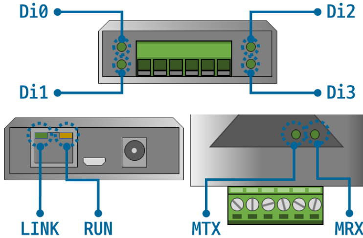
그림 1-10 LED
