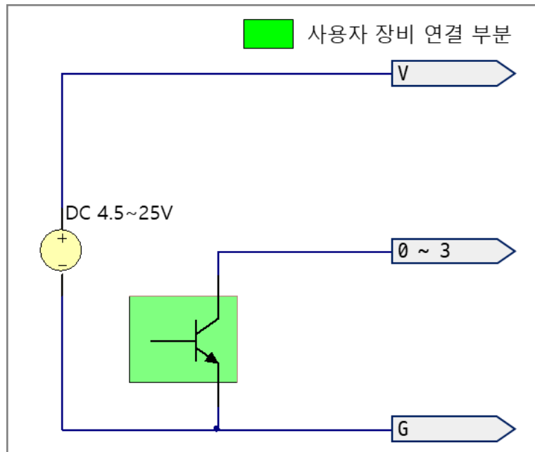
그림 1-8 NPN 트랜지스터 연결
