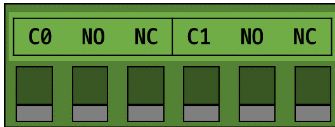
그림 1-4 디지털 출력 포트
