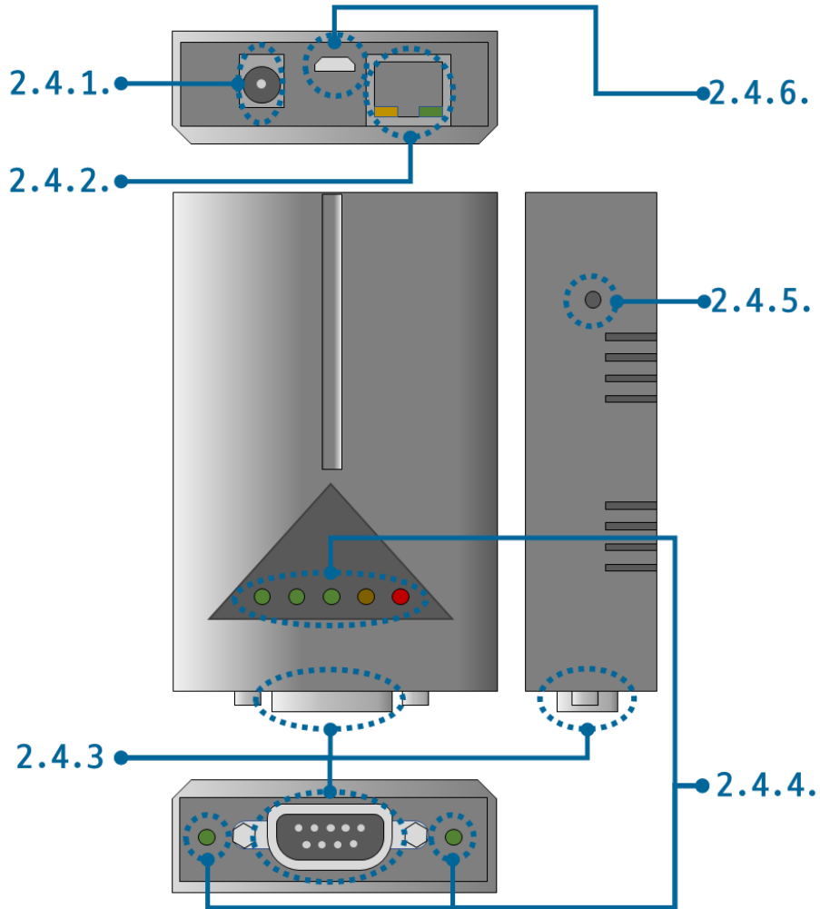
그림 2-1 인터페이스
