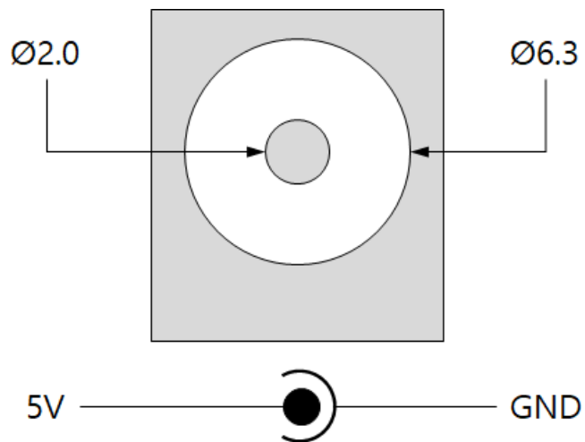
그림 2-2 전원 부
