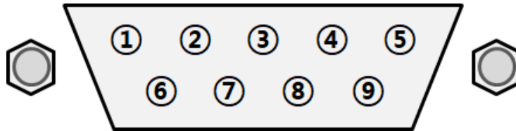
그림 2-4 시리얼포트 인터페이스
