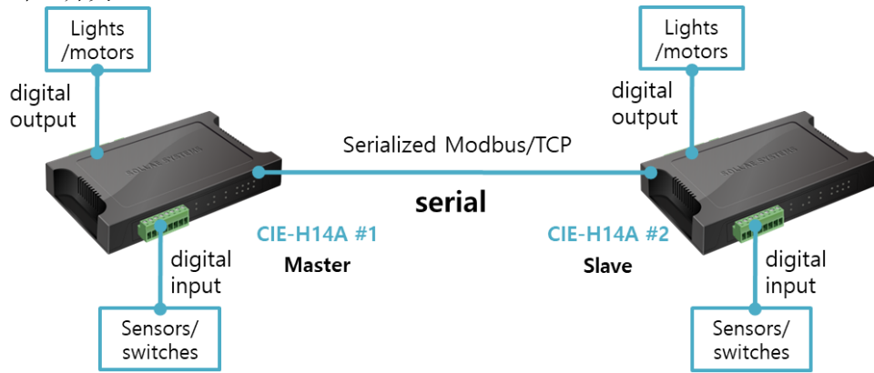
图 1-4 串口开关
