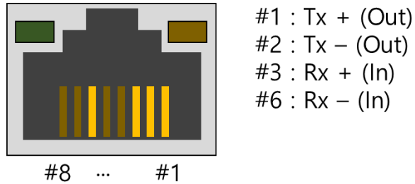
图 1-13 RJ45以太网连接器规格
