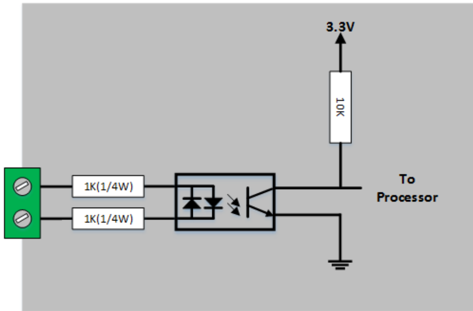
图 1-9 输入端口 电路图
