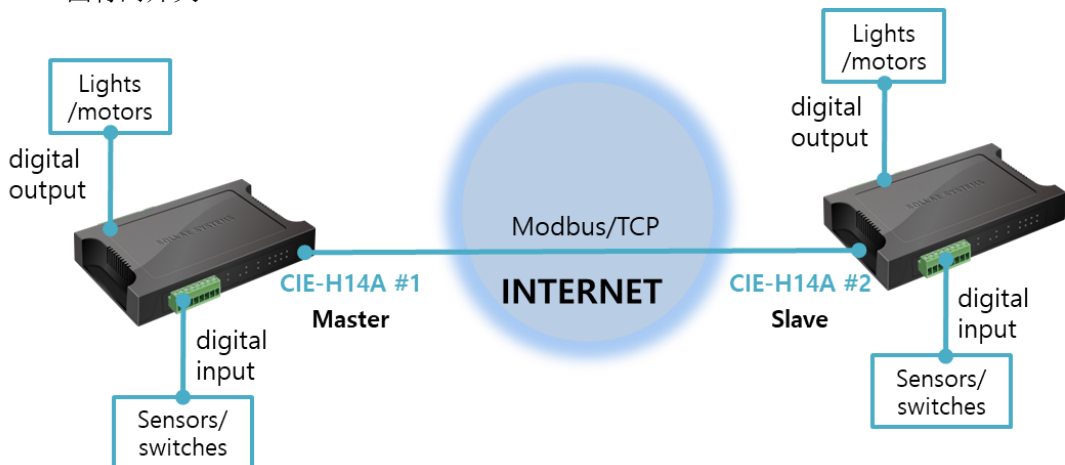
图 1-3 因特网网关
