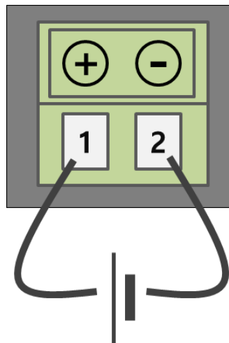
图 1-8 电源输入方式
