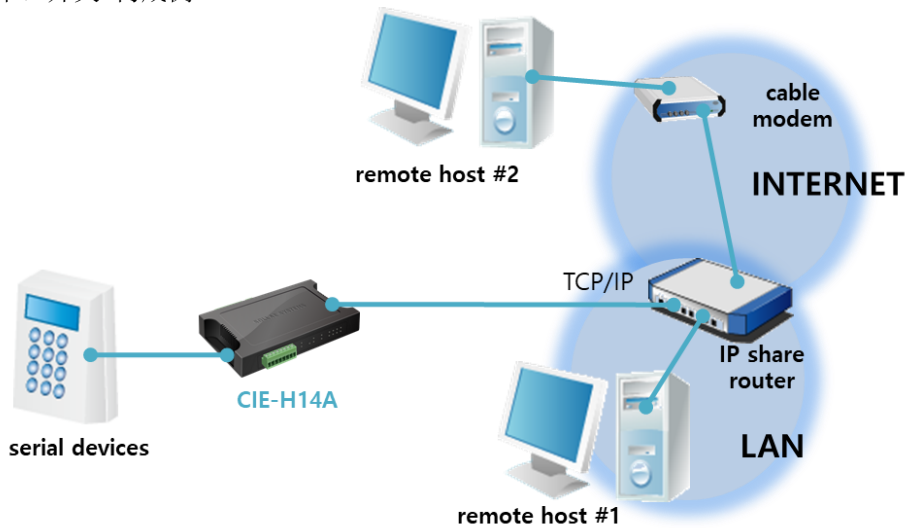
图 1-6 串口设备服务器
