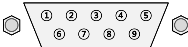
图 1-12 D-sub Male连接器
