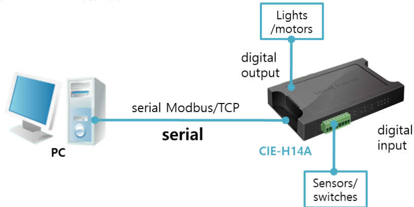
图 1-2 串口 Modbus/TCP构成 例
