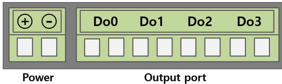
图 1-7 CIE-H14A输出端口
