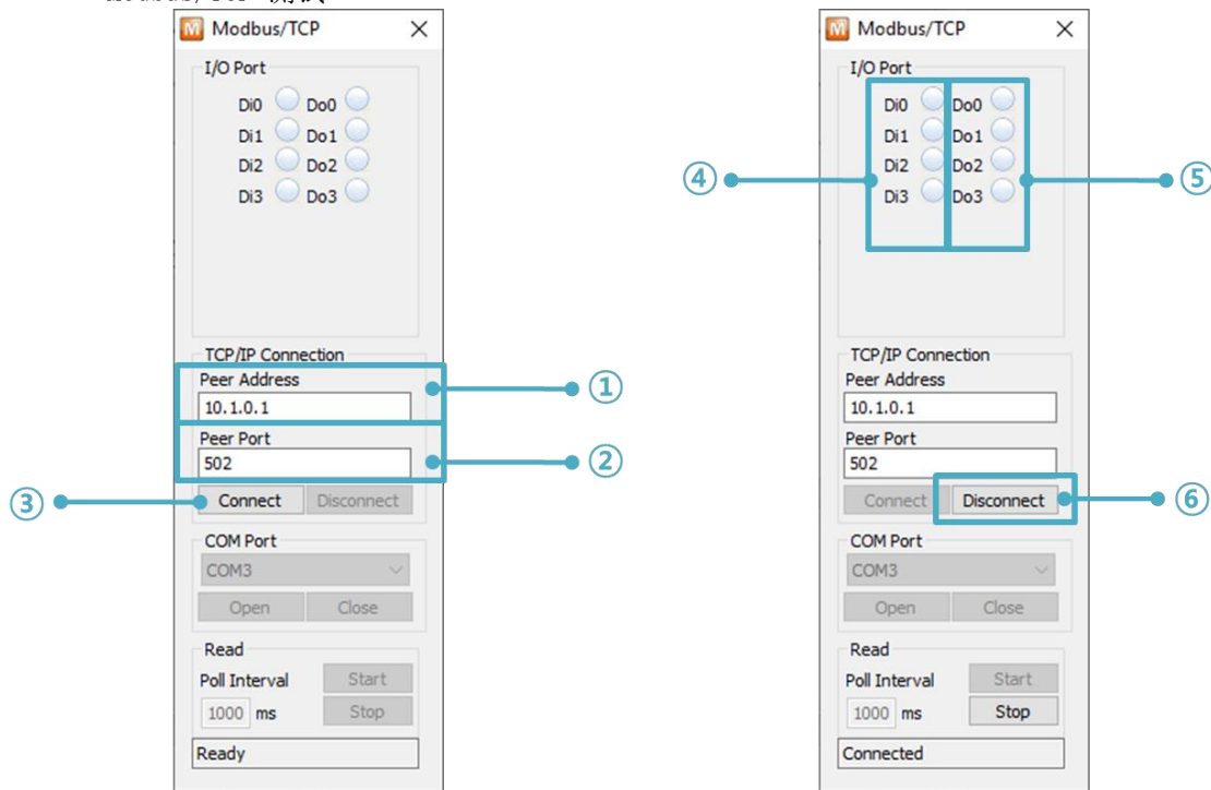
图 2-4 Modbus/TCP 测试
