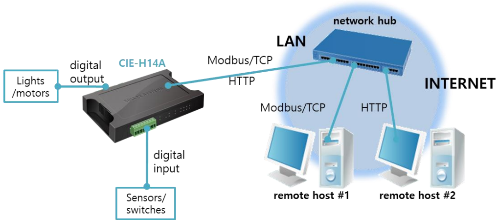
图 1-1 远程I/O设备构成 例
