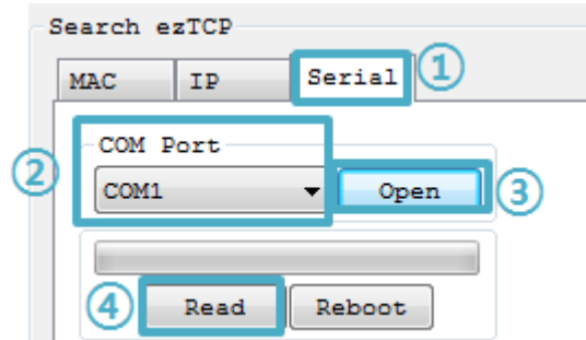
图 2-8 通过串行端口读取参数值
