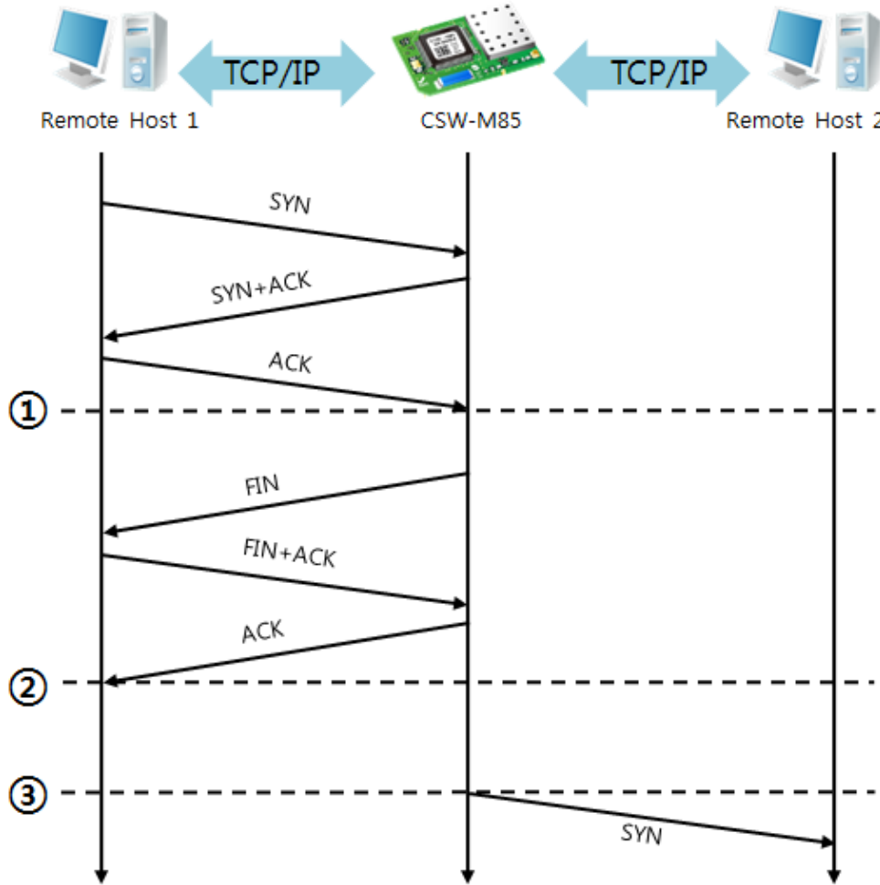
图 5-6 TCP 服务器/客户端模式的情况
