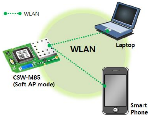
图 2-5 Soft AP模式
