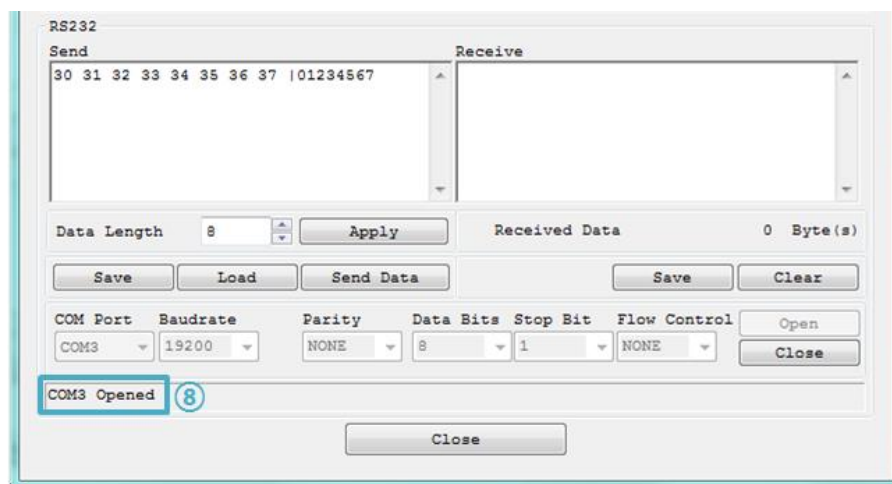
图 2-15 确认打开COM端口
