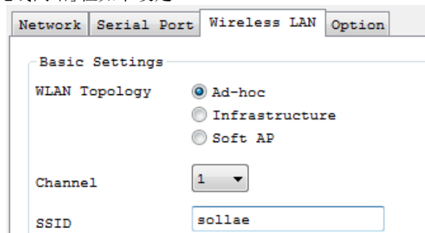
图 2-4 Ad-hoc模式设定
