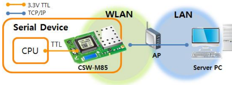
图 1-2 利用AP的内部网络连接
