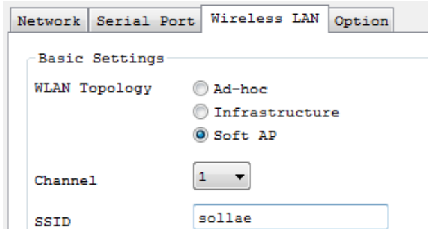
图 2-6 Soft AP模式设定
