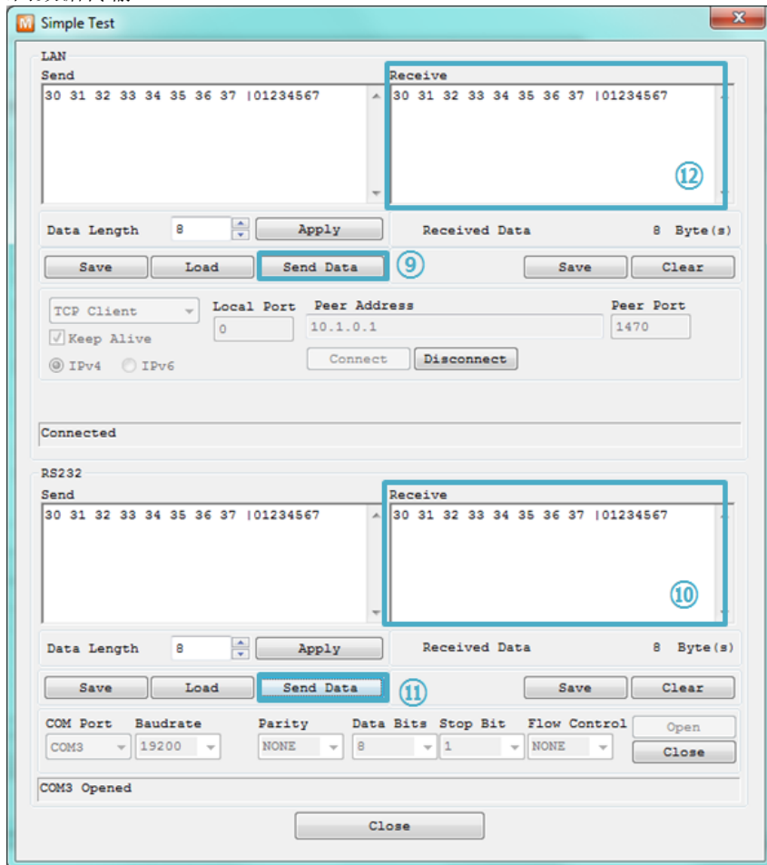
图 2-16 正常的的数据传送
