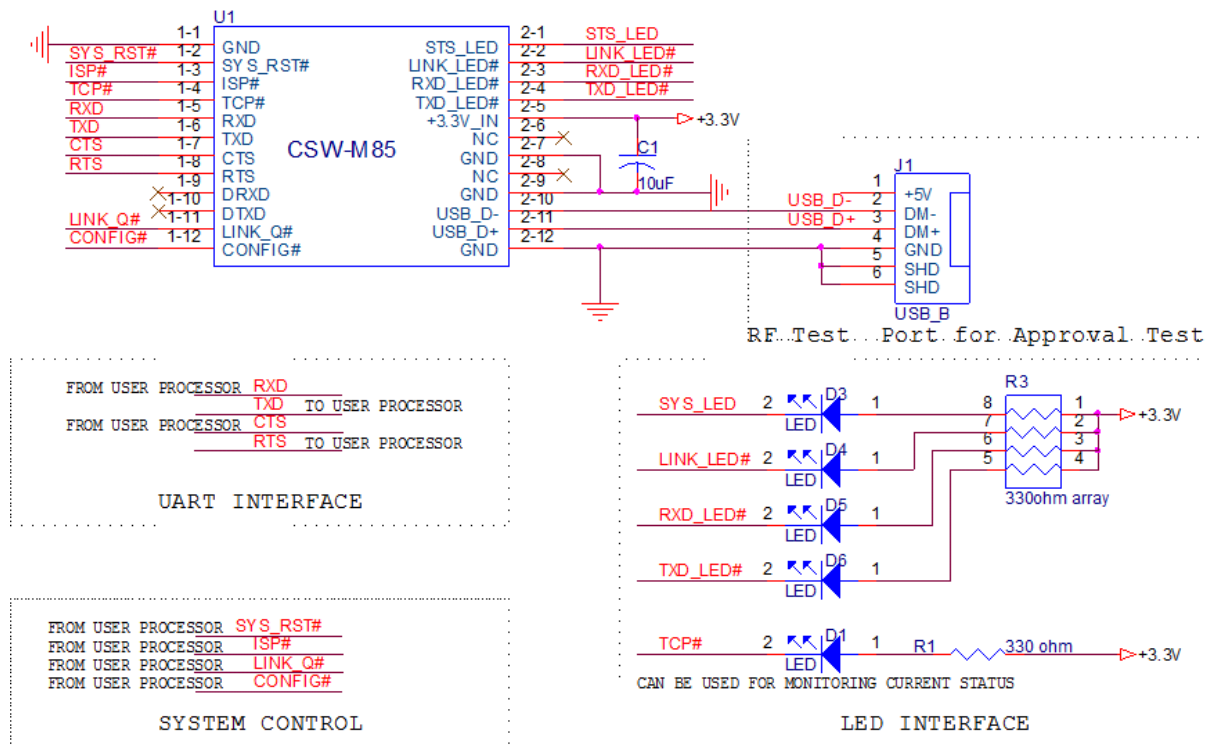
图 1-6 应用电路图
