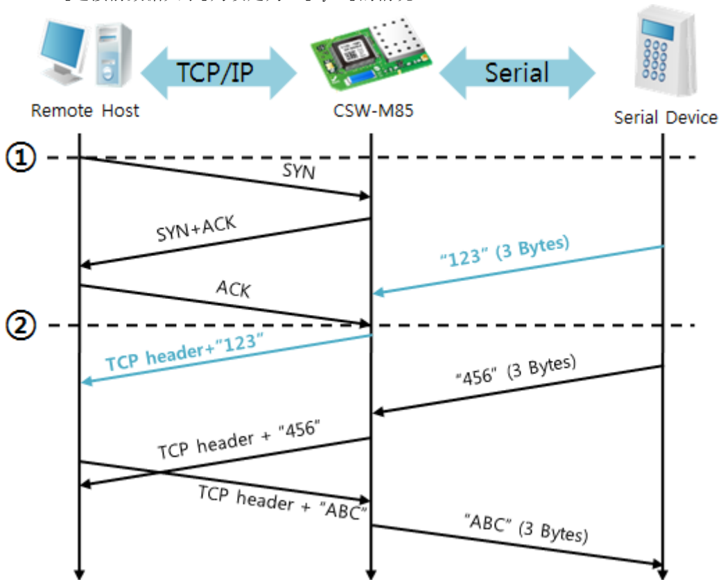
图 5-2 连接前数据大小为1的情况
