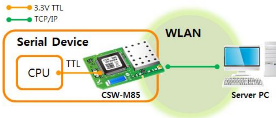
图 1-1 可进行无线连接PC构成1:1网络
