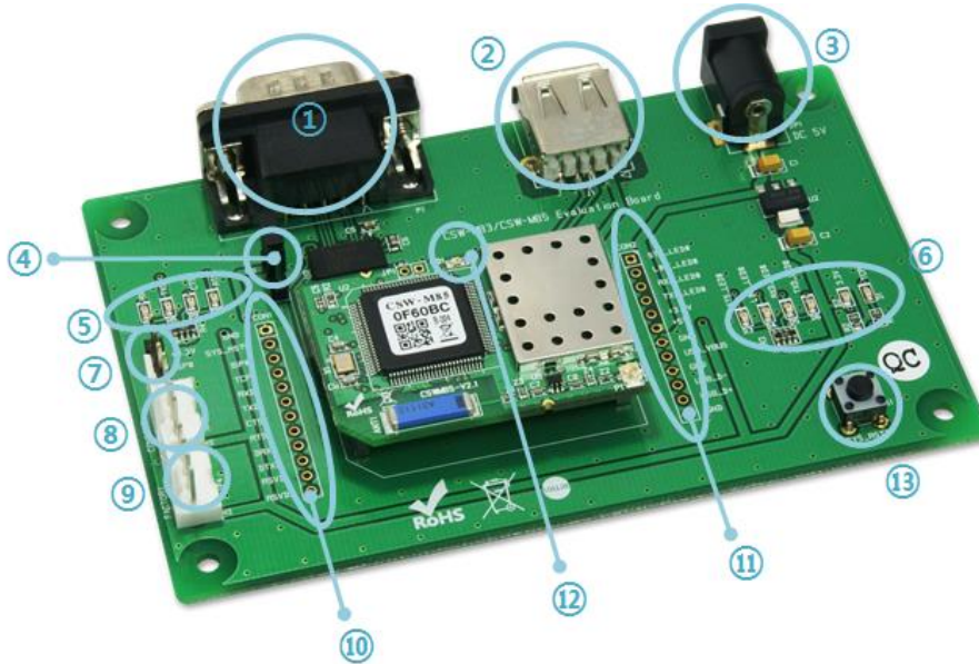
图 1-7 开发用测试板
