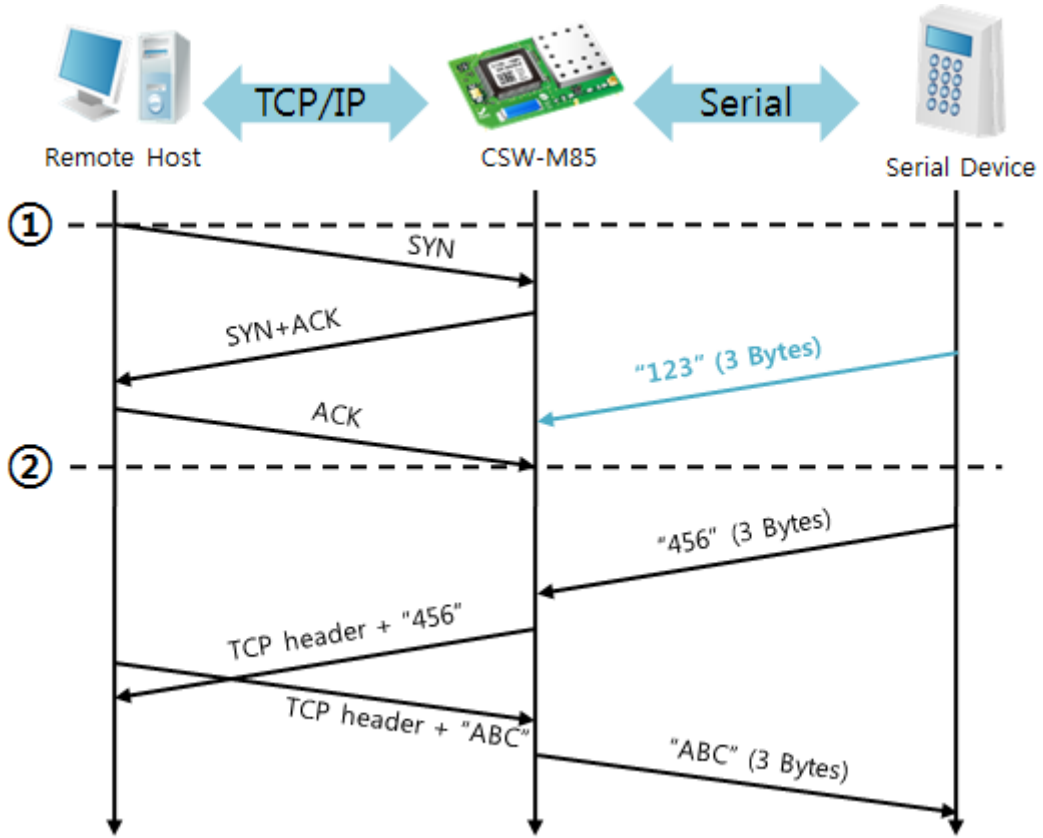
图 5-1 连接前数据代谢大小为0的情况
