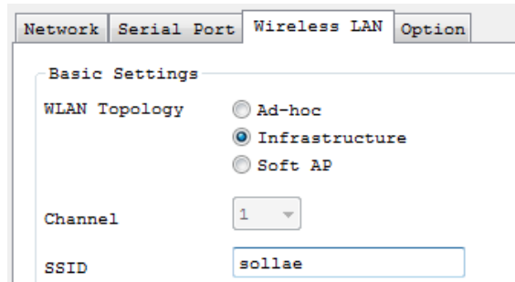
图 2-2 Infrastructure设定
