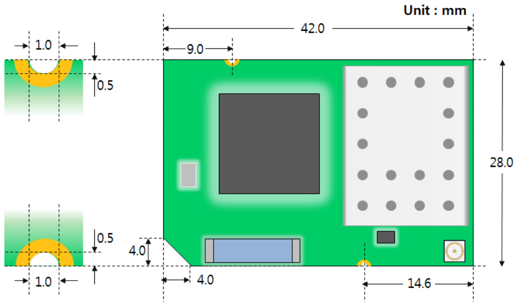
图 1-4 CSW-M85 规格 (Top view)
