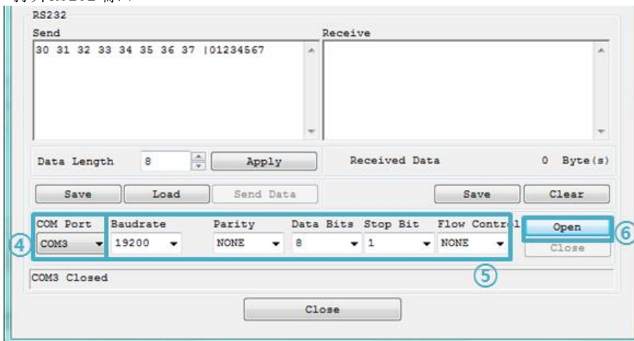
图 2-13 通过串行打开COM端口
