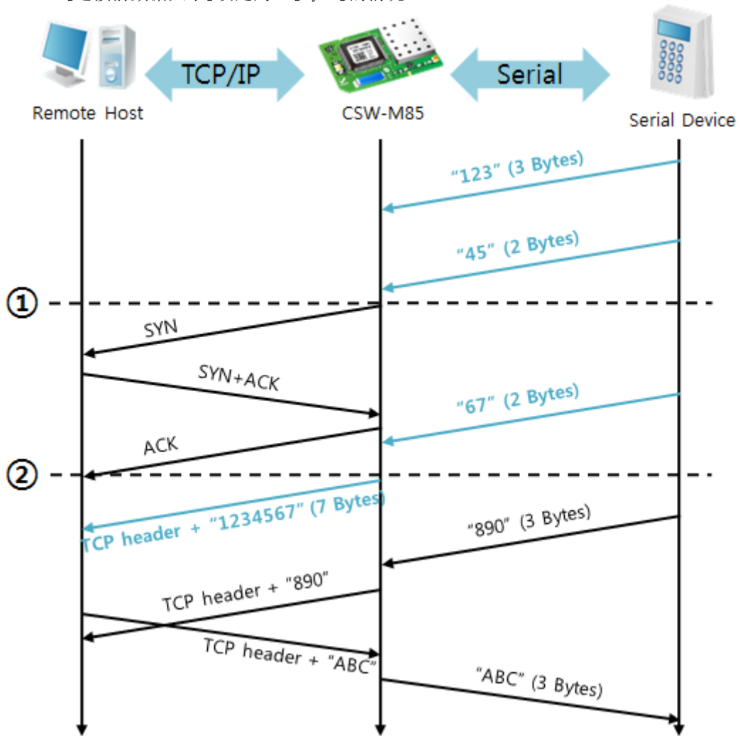
图 5-5 连接前数据大小为1的情况
