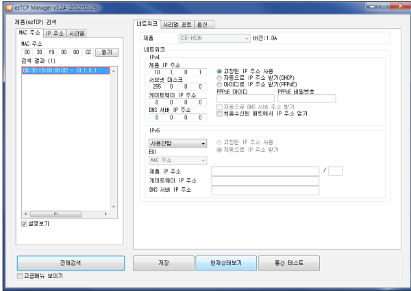
[ezManager 실행화면]
