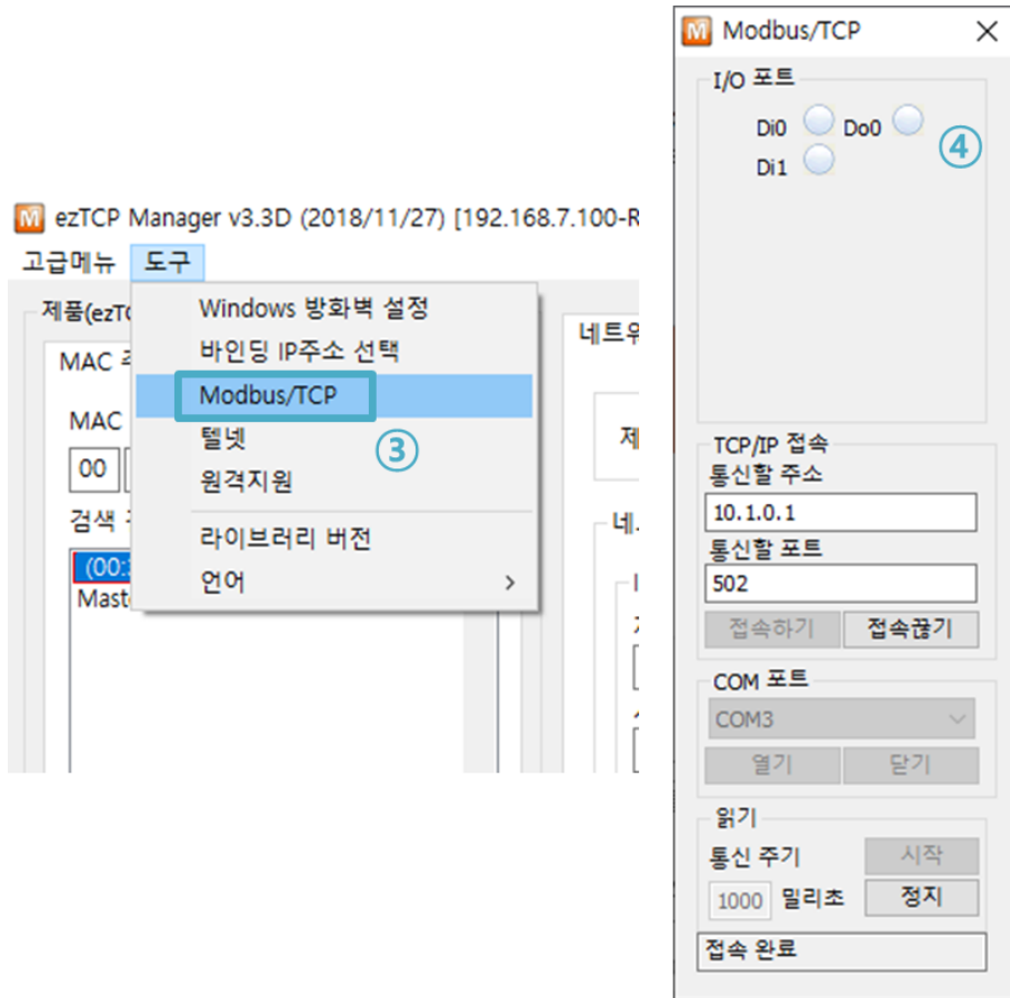
그림 2-3 Modbus/TCP 통신 테스트 프로그램
