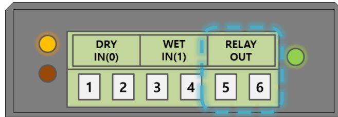
그림 1-8 출력포트 (정면 패널)
