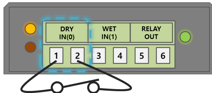
그림 1-5 접점입력 방식
