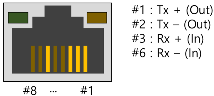
그림 1-10 RJ45 이더넷 커넥터 사양
