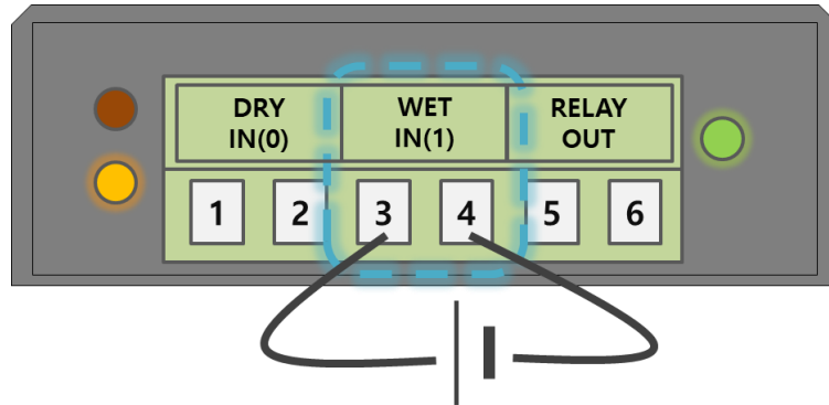
그림 1-6 전압입력 방식
