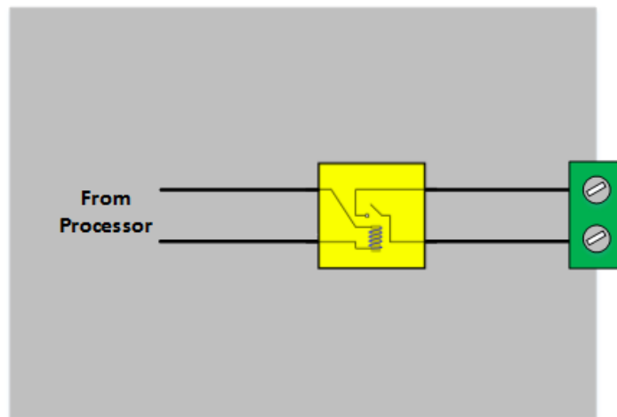
그림 1-9 출력포트 회로도
