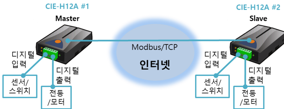
그림 1-2 인터넷 스위치 구성 예
