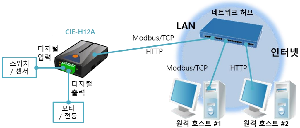
그림 1-1 원격 디지털 입/출력 감시/제어 구성 예
