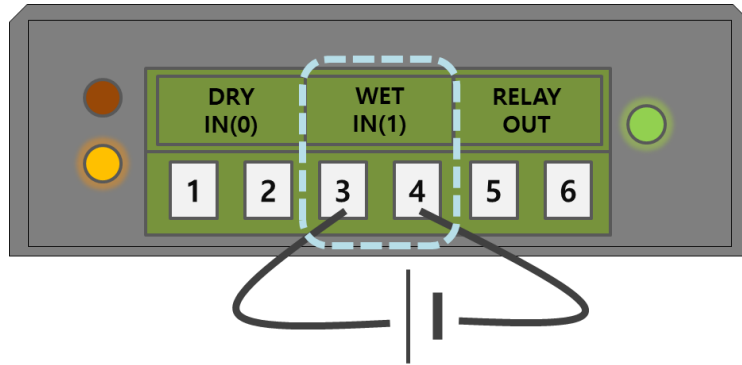
그림 1-5 WET IN 포트
