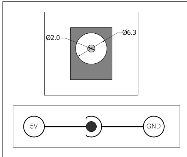
그림 1-10 전원 부
