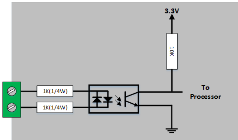
그림 1-6 WET IN 포트 회로도
