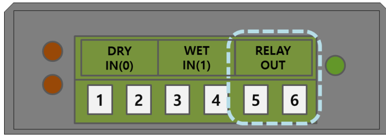
그림 1-7 출력 포트
