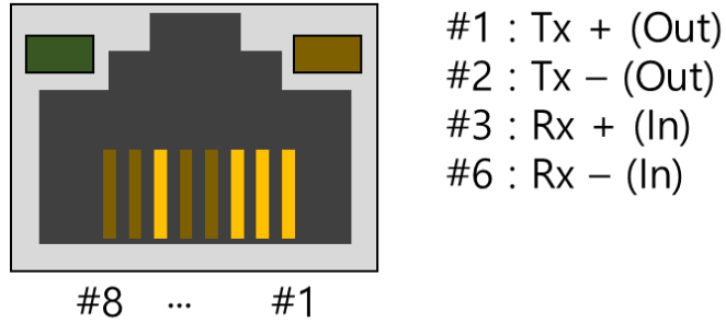
그림 1-9 이더넷 커넥터
