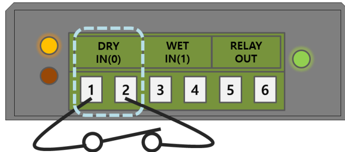
그림 1-4 DRY IN 포트
