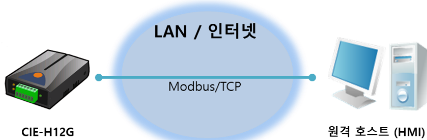
그림 1-1 원격 호스트(HMI)와 1:1 구성
