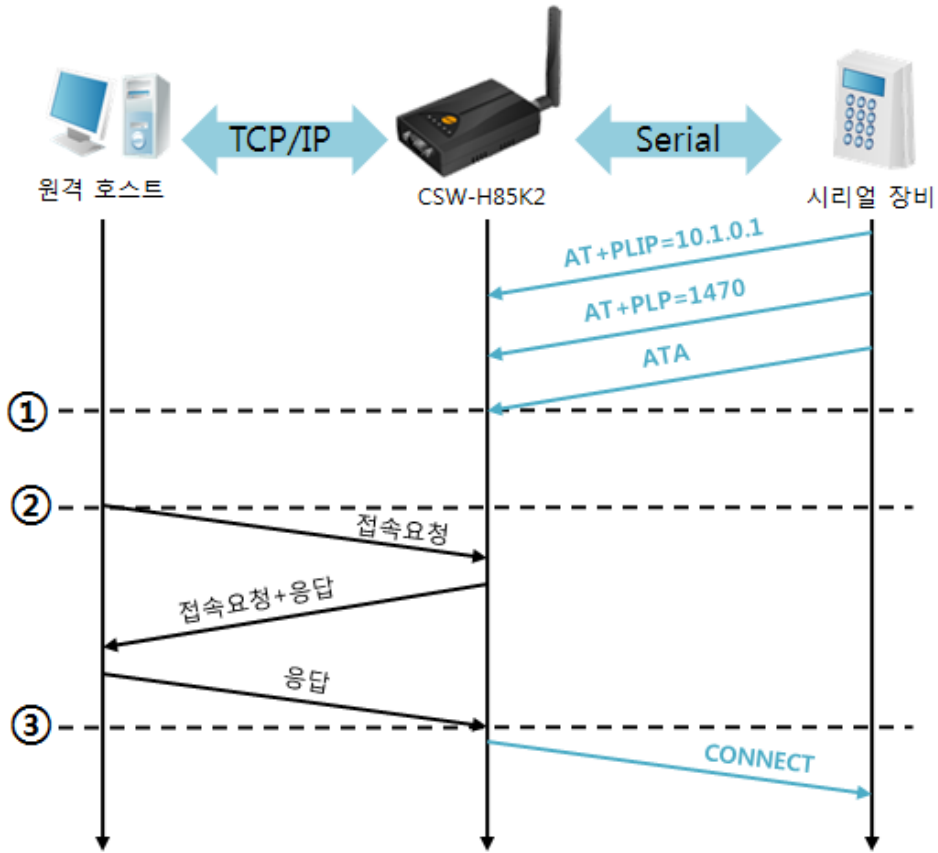
그림 5-7 TCP 수동접속
