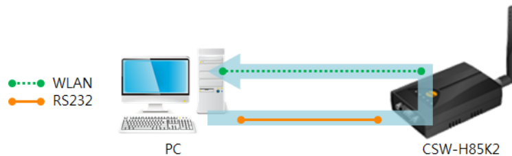
그림 2-19 RS232 → WLAN
