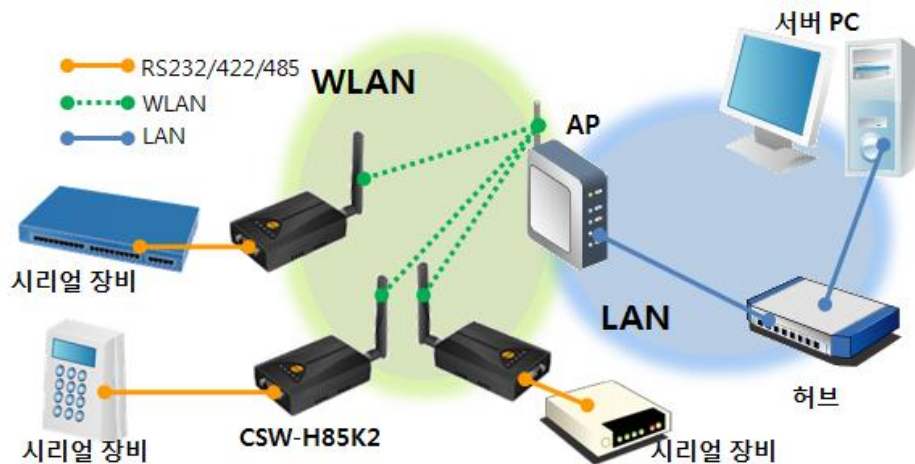
그림 2-1 인프라스트럭처 모드
