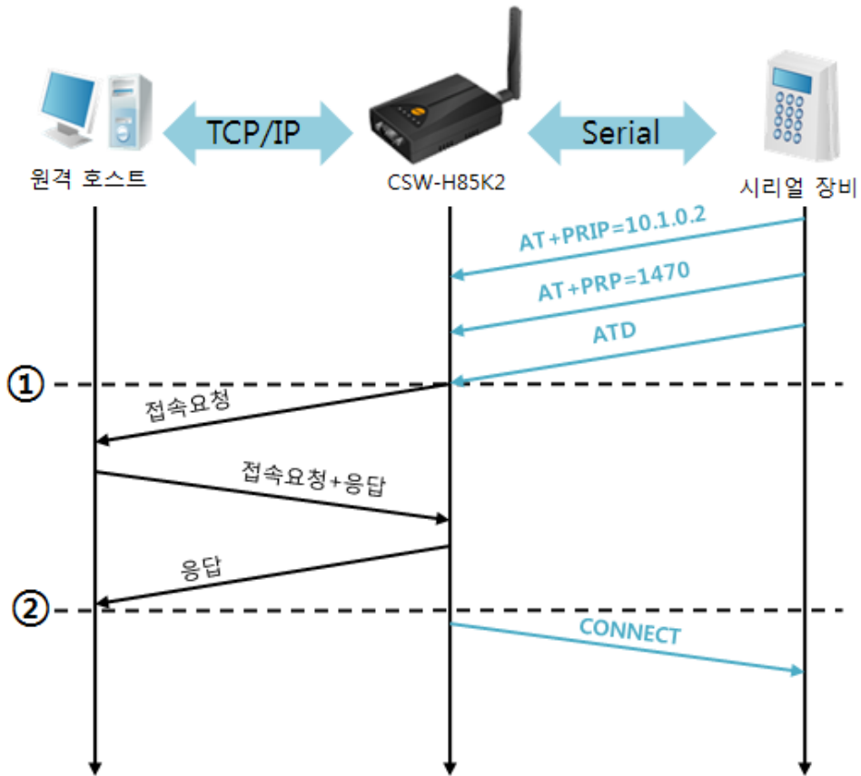
그림 5-8 TCP 능동접속
