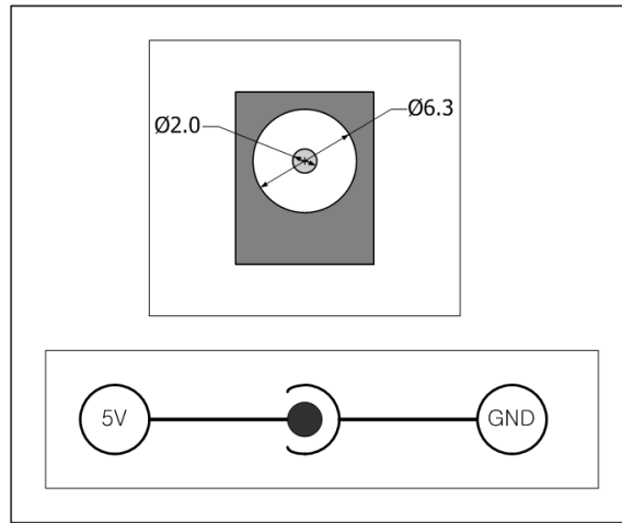
그림 1-8 전원 부
