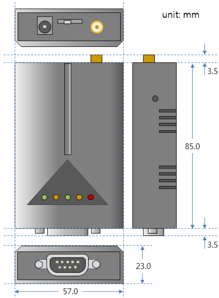
그림 1-4 CSW-H85K2 치수
