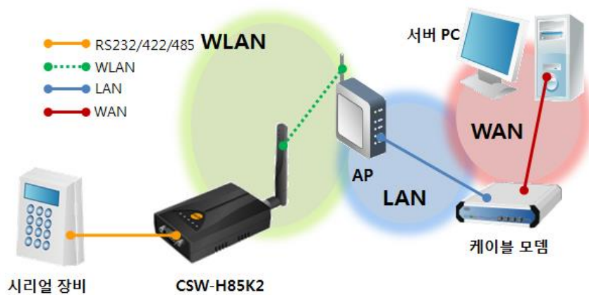
그림 1-3 xDSL/케이블 모뎀을 이용한 인터넷 연결
