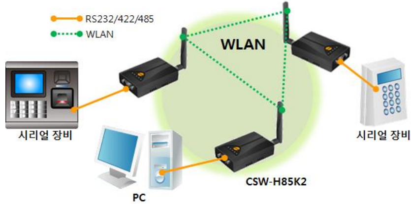
그림 2-3 애드혹 모드
