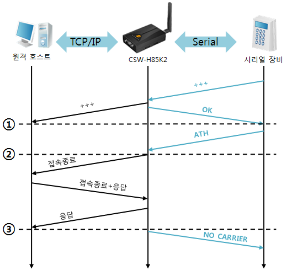
그림 5-9 TCP 접속종료
